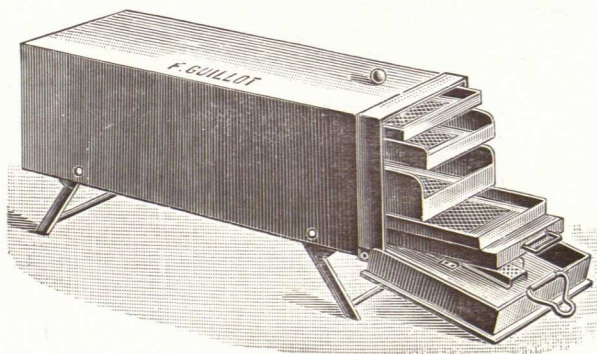
K. 39. Etuve du Docteur Gross pour la stérilisation des instruments, gants, pansements, par les vapeurs de trioxyméthylène.
