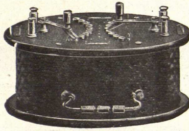
B. 1206. Boîte ovale pour cautère et lumière sur alternatif. réglage par 2 manettes à plots. Usage simultané du cautère et de la lumière ..... 260 »
