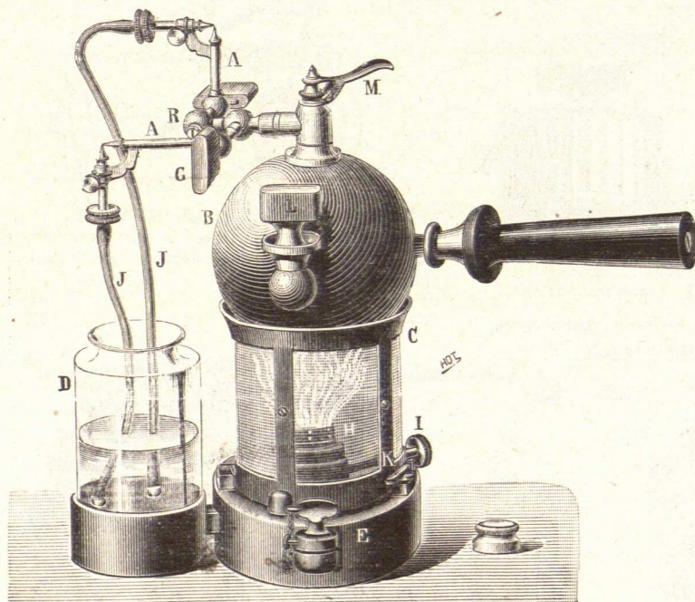
B. 762. Pulvérisateur de Lucas Championnière, grand modèle des hôpitaux à 2 becs, marchant 2 heures ..... 190 »
