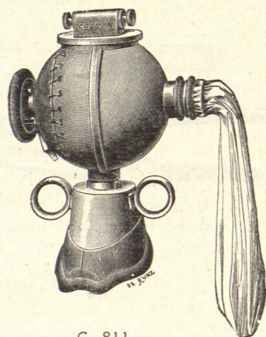
C. 811. Appareil à éther du D r Ombredanne, complet en boîte..... 455 »
