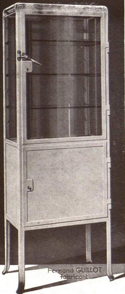
L. 330. Vitrine à instruments ; coffre en tôle contenant une étagère ; contour de la partie supérieure en verre double ; serrure ; poignée nickelée ; trois étagères en glace ; haut. 1 m. 70, larg. 0 m. 60, prof. 0 m. 35 ..... 975 »
