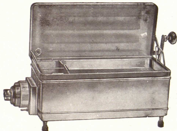
K. 84. Stérilisateur électrique, dernier modèle, avec couvercle à charnières, ouverture par levier, commutateur à 3 intensités, pour la stérilisation par ébullition ou air chaud. Dimensions : 280x130x80 . . . . 350 »
