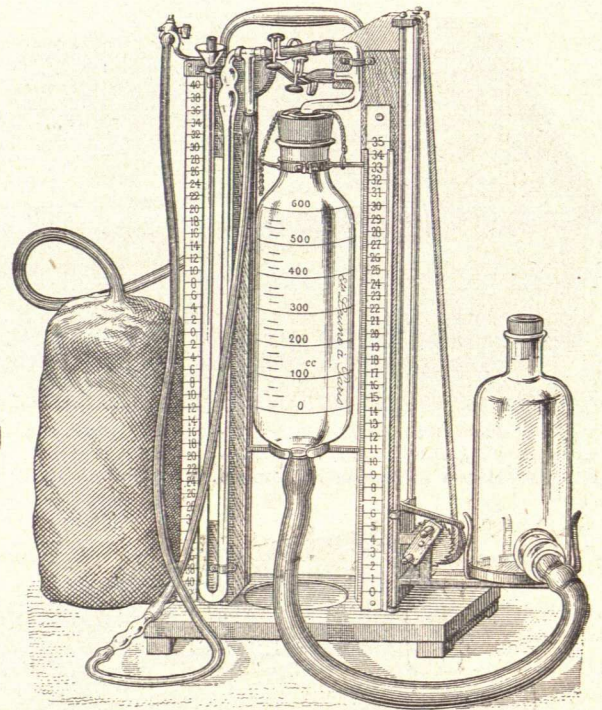
B. 600. Appareil à pneumothorax du D r Kuss, grand modèle pour Cliniques et Hôpitaux, complet en ordre de marche ..... 1.185 »
