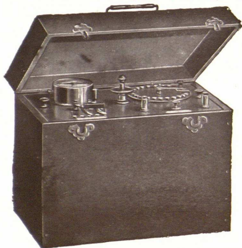
M. 450. Appareil à pile au bisulfate de mercure, monté avec galvanomètre, inverseur, interrupteur, avec charge, cordons, accessoires.
