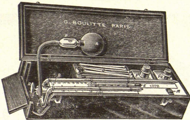
A. 84. Viscosimètre du Prof. W. Hess pour la mesure de la viscosité sanguine ..... 220 »
