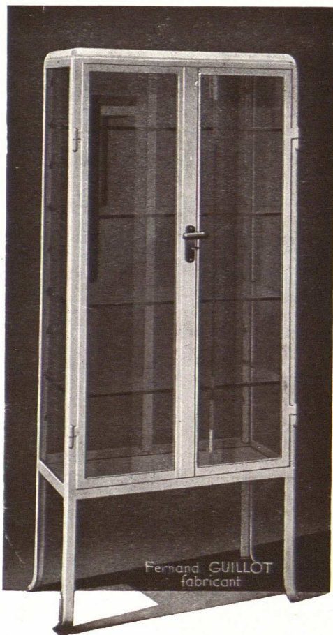
L. 324. Vitrine à instruments. Grand modèle à 2 portes. Cadre en fer cornière et dessus en tôle formant dôme ; contour en verre double ; deux portes à fermeture hermétique par crémone ; fond en verre martelé. Quatre tablettes intérieures en glace claire rodée et polie, se posant sur crémaillère réglables en hauteur. Dimensions : haut. 1 m 70 ; larg. 0 m 75 ; prof. 0 m 40 .. 1.075 »
